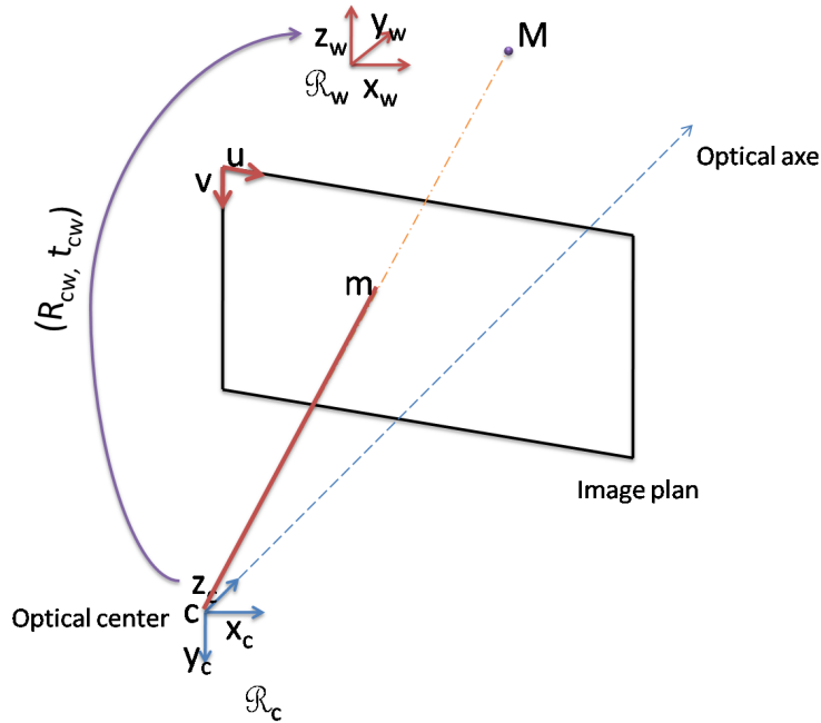
FIGURE A.1: Modèle de projection perspective : modèle sténopé
