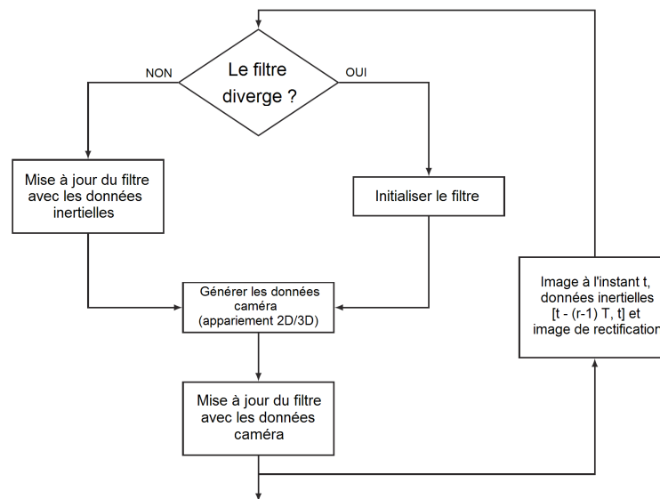
FIGURE 3.6: Flot de données dans l'approche de localisation proposée dans [Bleser, 2009]
