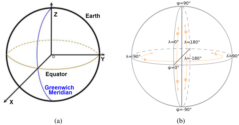
FIGURE 4.12: (a) repère défini par le système WGS84 (b) Coordonnées géographiques : longitude et latitude
