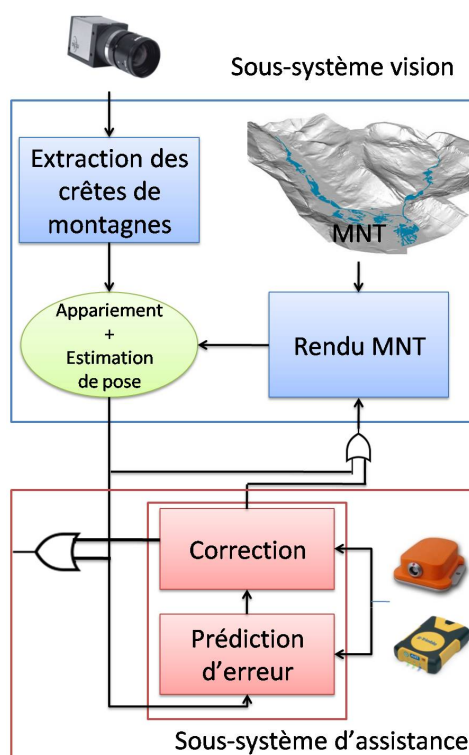
FIGURE D.1: Système multi-capteur pour la localisation en environnement panoramique
