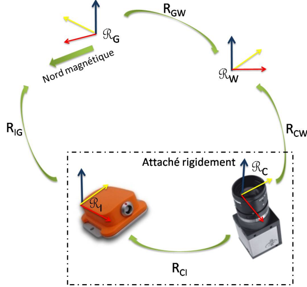
FIGURE 4.10: Configuration des repères
