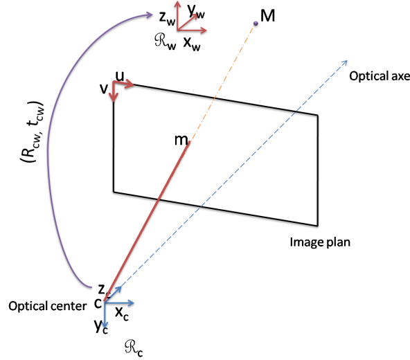
FIGURE 2.12: Modèle de caméra sténopé
