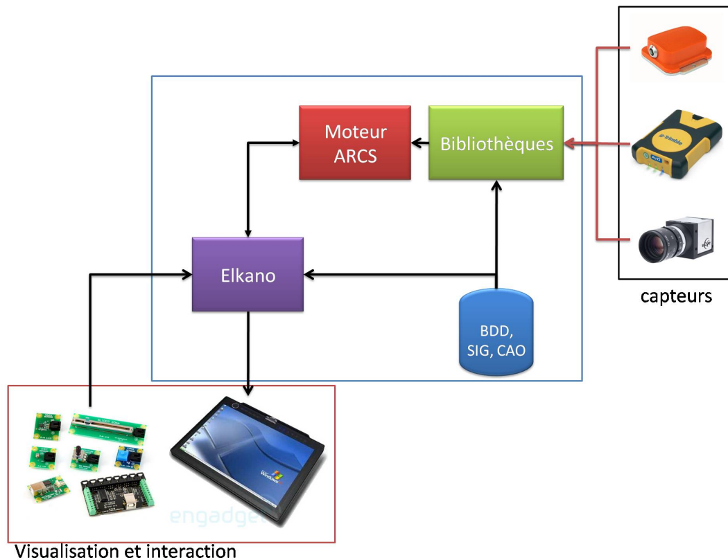
FIGURE 5.23: Flot de données dans la plateforme RAXENV
