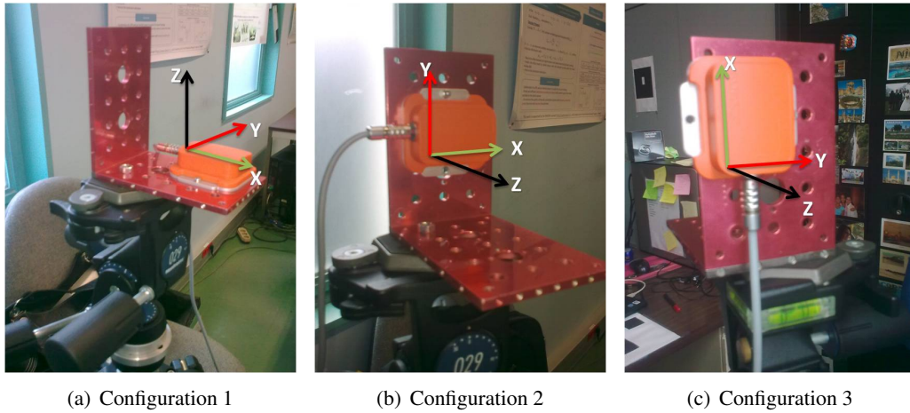
FIGURE 4.15: Les différentes configurations pour la précision des orientations de la centrale inertielle
