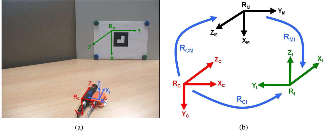
FIGURE 4.7: (a) Représentation des repères utilisés (b) Représentation des rotations entre les repères utilisés dans [Maidi et al., 2009]
