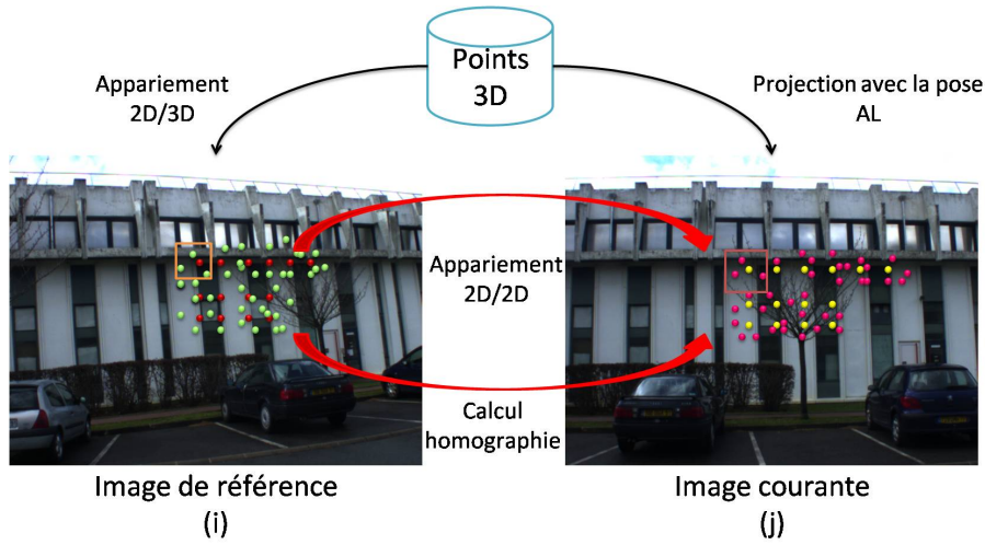
FIGURE 5.4: Réinitialisation automatique : schéma illustratif
