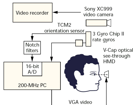
FIGURE 3.1: Descriptif du système multi-capteurs présenté dans [You et al., 1999]
