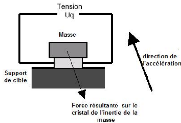
FIGURE 1.8: Schéma de principe d'un accéléromètre
