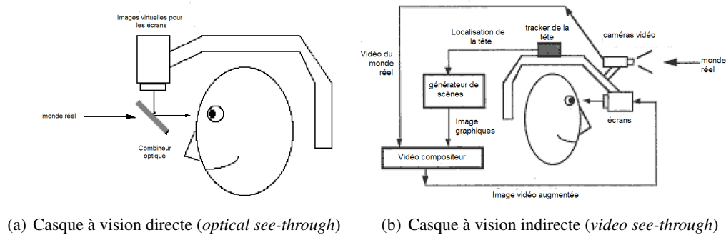
FIGURE 1.13: Classification des casques HMD pour la RA selon [Azuma, 1997]
