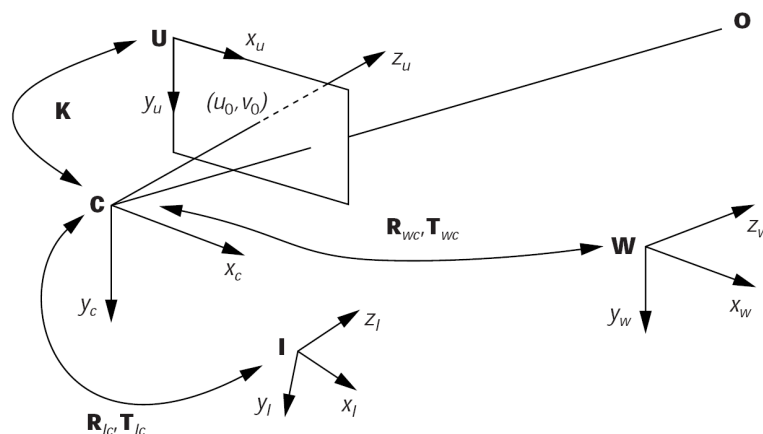
FIGURE 4.1: Configuration des systèmes de coordonnées utilisés dans le capteur hybride proposé par [You et al., 1999]
