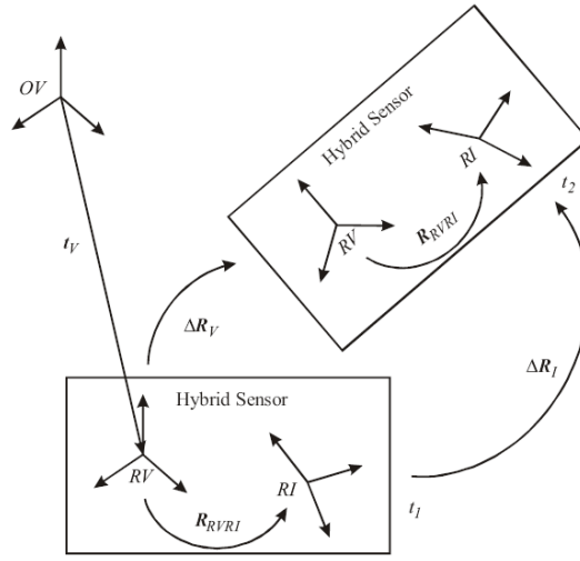
FIGURE 4.3: Approche de calibration décrite par [Lang et Pinz, 2005]
