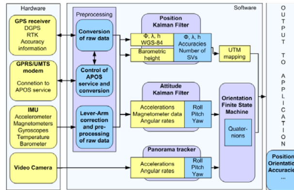
FIGURE 3.12: Architecture du système proposé dans [Schall et al., 2009]
