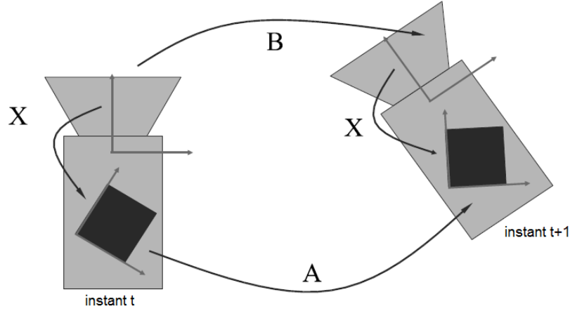
FIGURE 4.5: Configuration utilisée dans [Aron et al., 2007] pour la calibration Hand-eye du capteur Inertiel/Caméra
