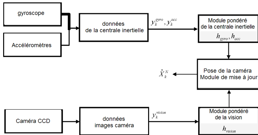
FIGURE 3.8: Un filtre complémentaire pour la fusion de capteurs [Ababsa et Mallem, 2007]
