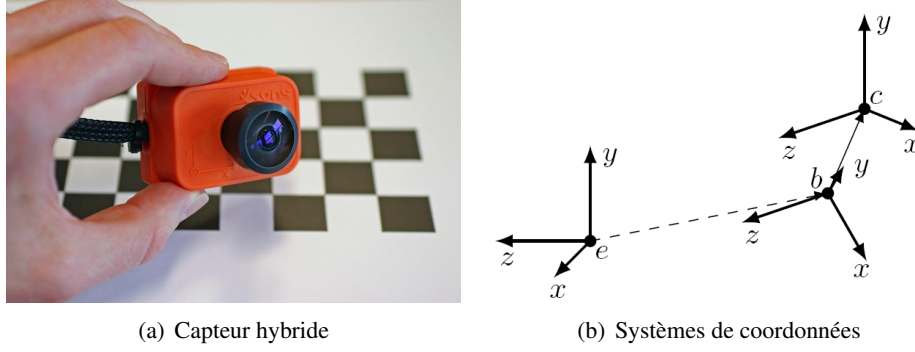
FIGURE 4.4: L'approche de Hol et al.
