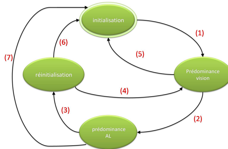
FIGURE 5.6: fonctionnement du système hybride de localisation
