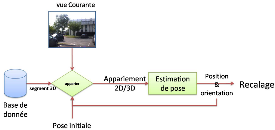
FIGURE C.1: Principe général de fonctionnement en utilisant une approche basée segment.
