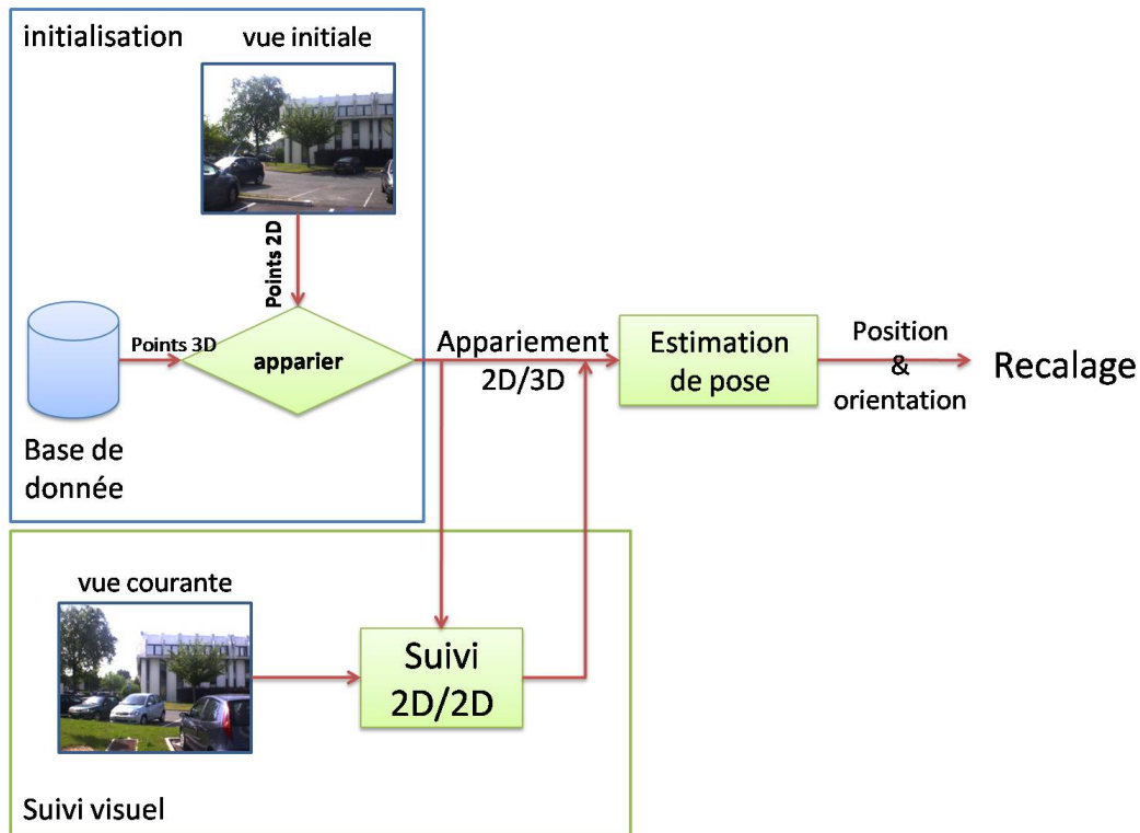
FIGURE 2.13: Principe général de fonctionnement en utilisant une approche basée points.
