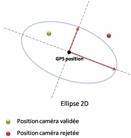
FIGURE 5.2: Intervalle de confiance défini pour valider les positions estimées par la caméra.
