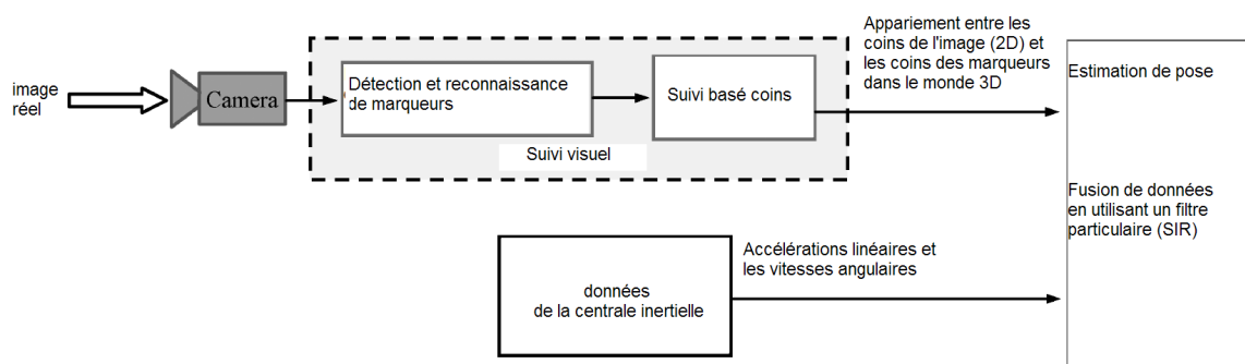
FIGURE 3.7: Le système Hybride proposé dans [Ababsa et Mallem, 2007] : flot de données
